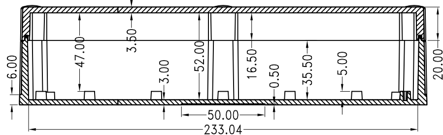
SEC: A-A
