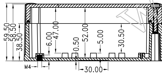
SEC: B-B
