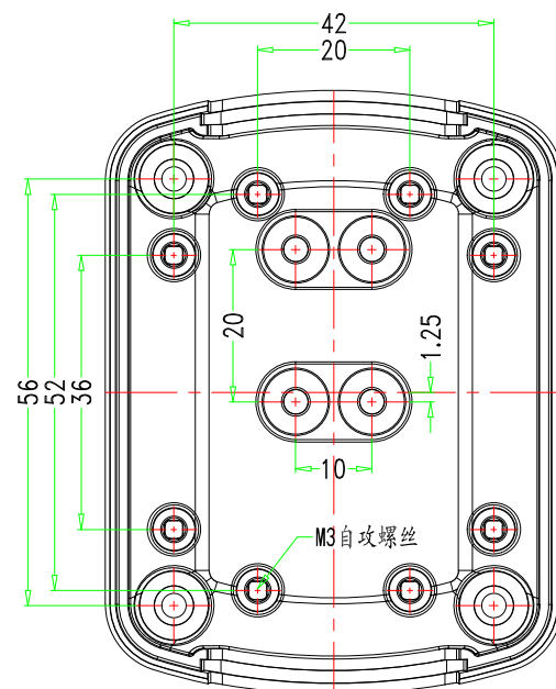
底壳内视图
