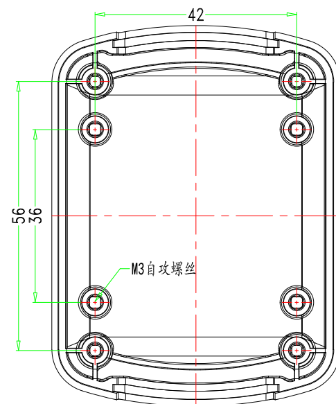
上壳内视图
