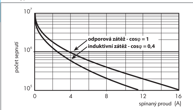
F 45 - elektrická životnost při AC typ 45.31...4310
