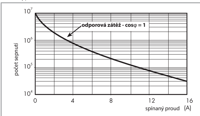
F 45 - elektrická životnost při AC typ 45.31/45.91
